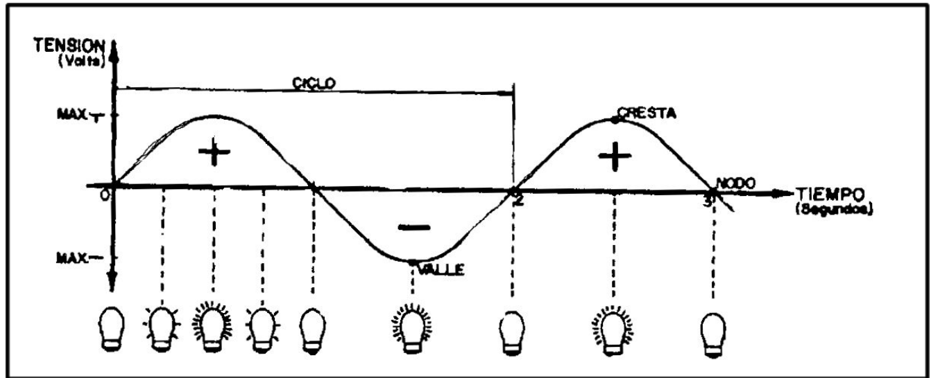
Gráfica de Corriente Alterna
